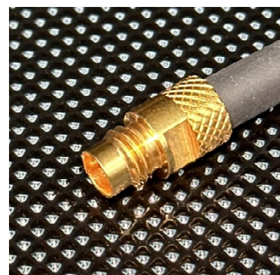
1/4-28UNF 4 pin plug
